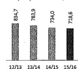
Frischwasserverbrauch in Liter je m 2 gewichteter Leiterplatte
