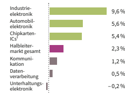
G 06 Durchschnittliche jährliche Wachstumsraten der wesentlichen Halbleiter-Zielmärkte im Zeitraum 2014 bis 2019
