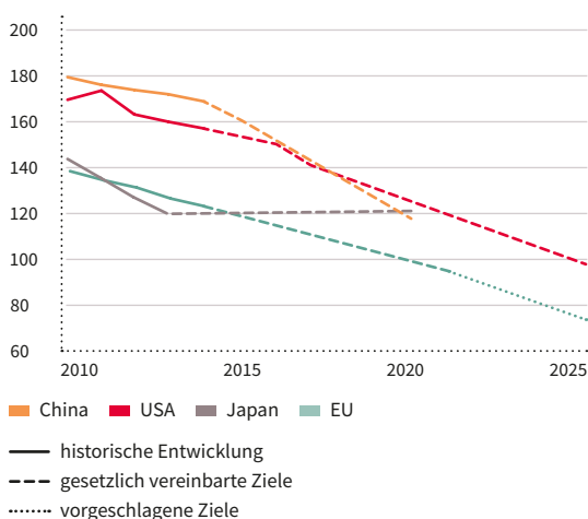
G 12 Gesetzlich vereinbarter Flottenausstoß der vier großen Automobilregionen CO 2 in Gramm pro Kilometer; normalisiert auf den NEDC Testzyklus
