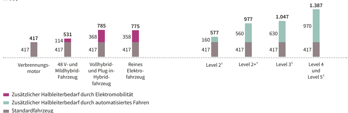
Zusätzlicher Halbleiterbedarf pro Fahrzeug durch Elektromobilität und automatisiertes Fahren in US$
